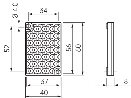
反光板 型号 (标配) : MQ40 / MQ40A
