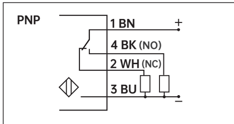
PNP 常开 (NO) + 常闭 (NC)
