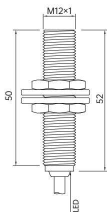
IS12...E1 尺寸图
