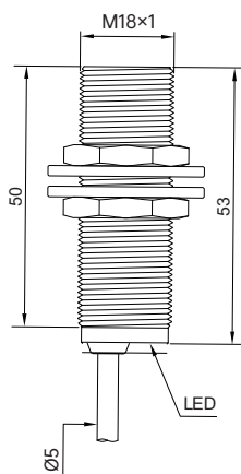
IS18...E1 尺寸图
