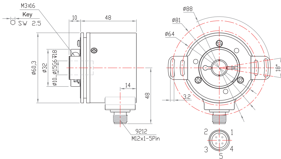
FDCE58B-CANopen+8138A
