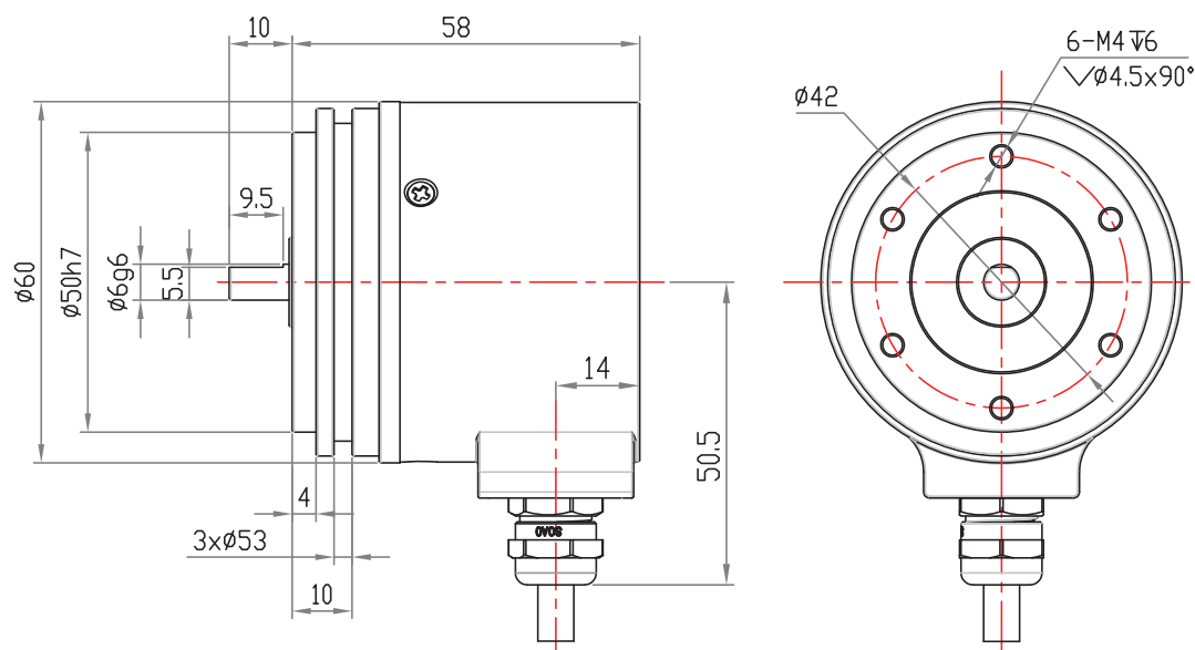
FDCE5804S-CANopen+9212
