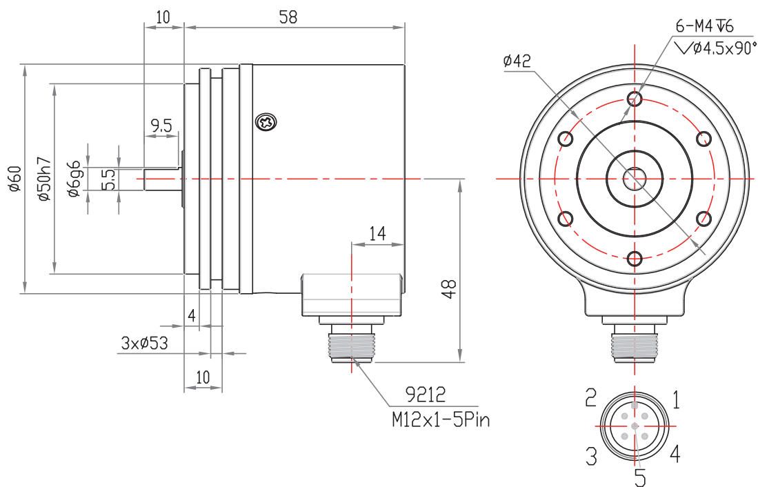
FDCE5804S-CANopen+9212
