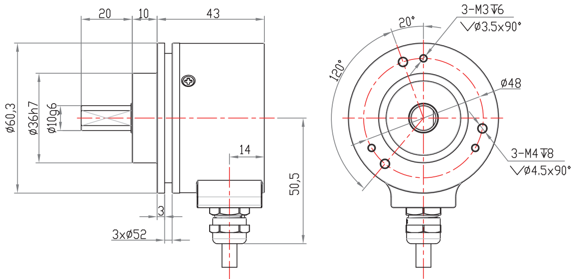
FDCE5803S-CANopen+9212
