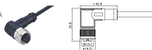
母头
