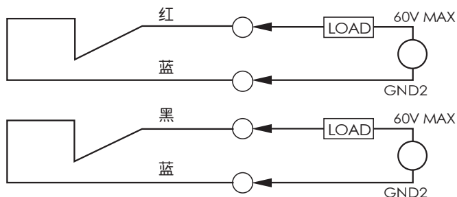
限位开关接线示意图:
